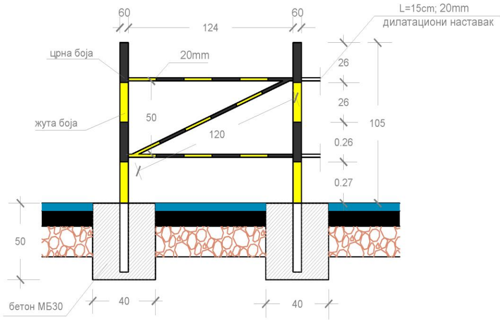
СКИЦА 1 ДЕТАЉ ПЕШАЧКЕ ОГРАДЕ
