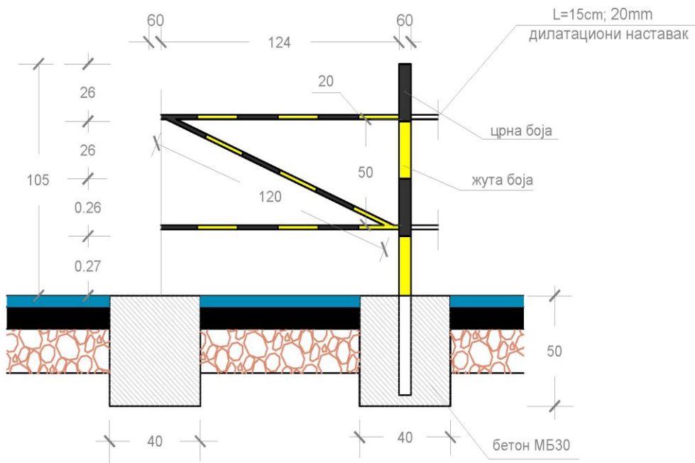
СКИЦА 2 ДЕТАЉ НАСТАВКА ПЕШАЧКЕ ОГРАДЕ
