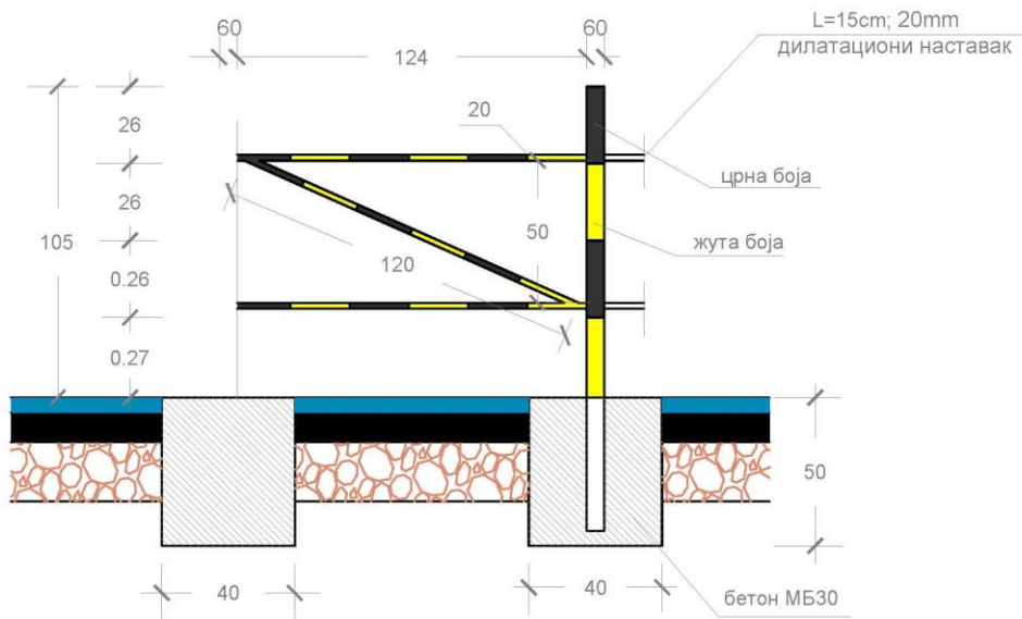
СКИЦА 2 ДЕТАЉ НАСТАВКА ПЕШАЧКЕ ОГРАДЕ
