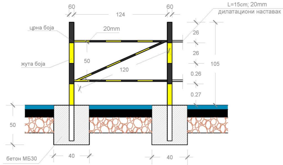
СКИЦА 1 ДЕТАЉ ПЕШАЧКЕ ОГРАДЕ
